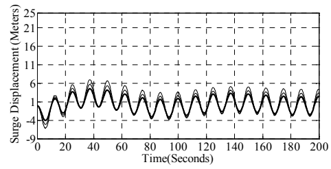
(d) wave period = 12.5 sec
